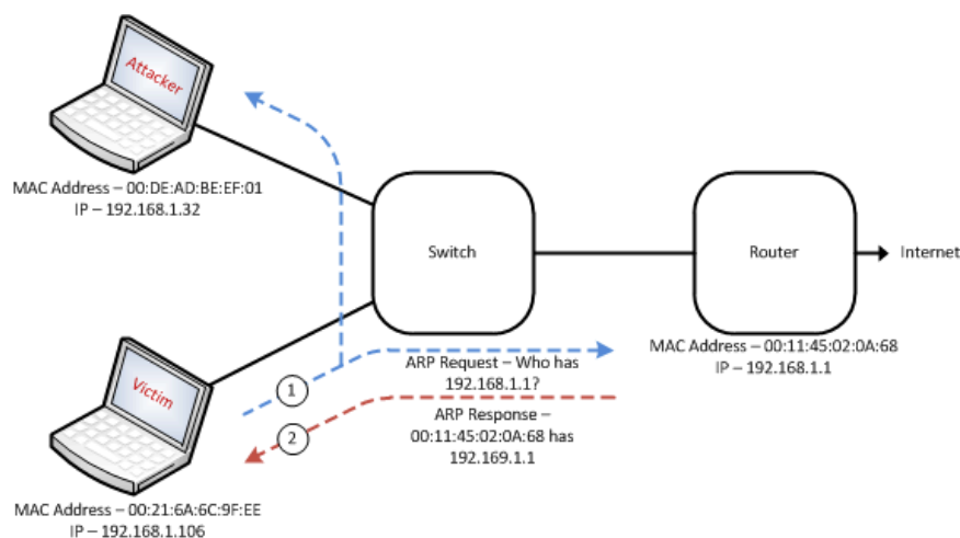
SLIKA 2: POTEK MITM-NAPADA. VIR: HTTP://WWW.SHORTESTPATHFIRST.NET
